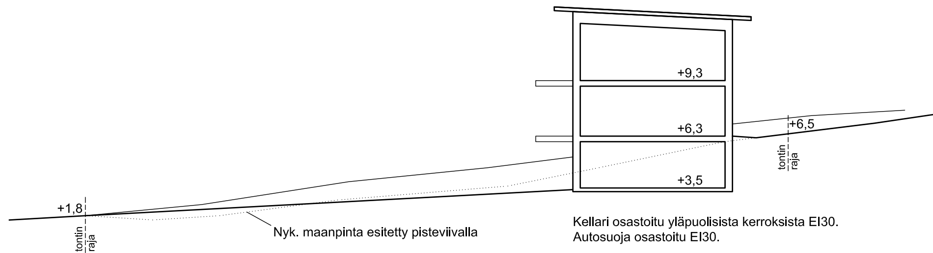
LEIKKAUS 1-1
