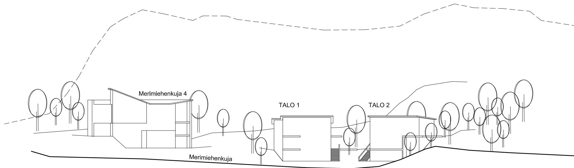
ALUELEIKKAUS MERIMIEHENKUJAA PITKIN, PROJEKTIOSUUNTA TALOA 1 KOHTI.
