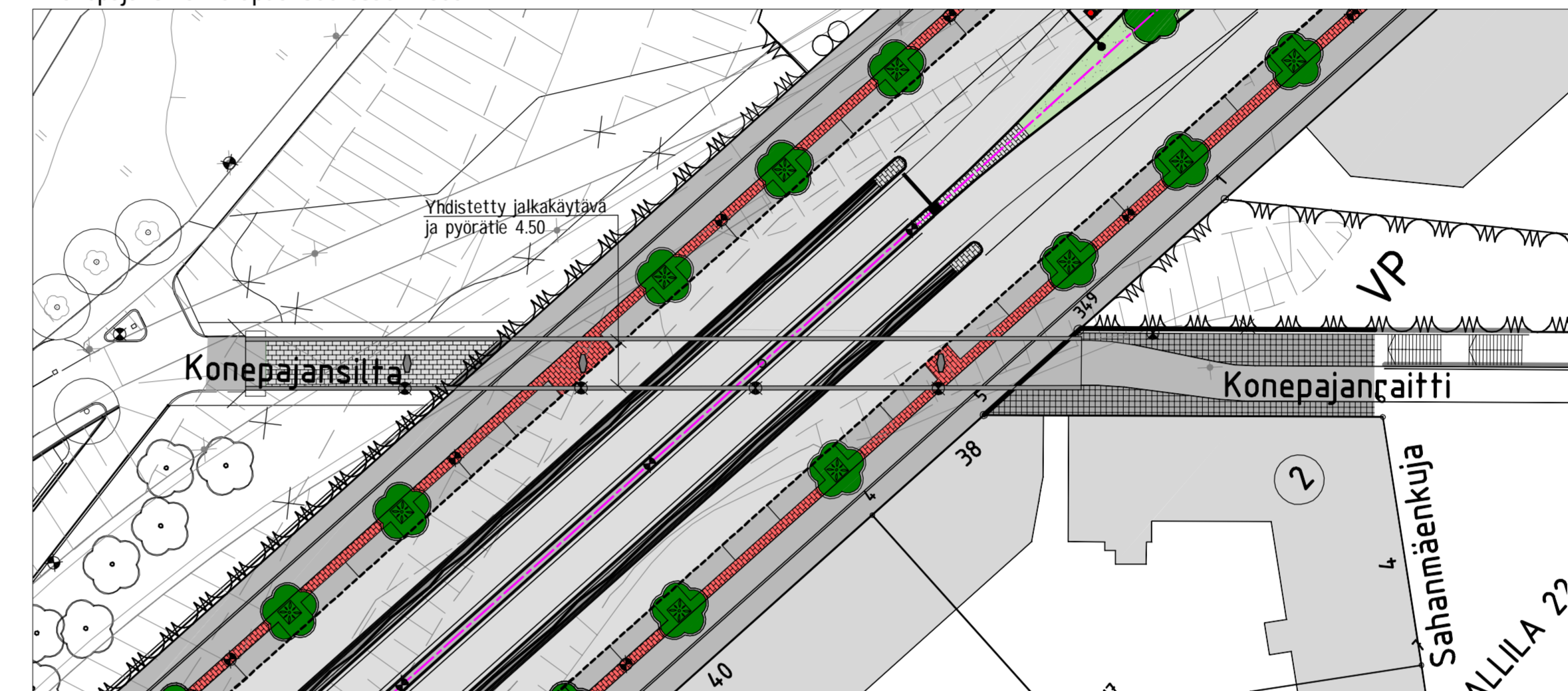
Konepajansillan alapuoliset osat 1:500
