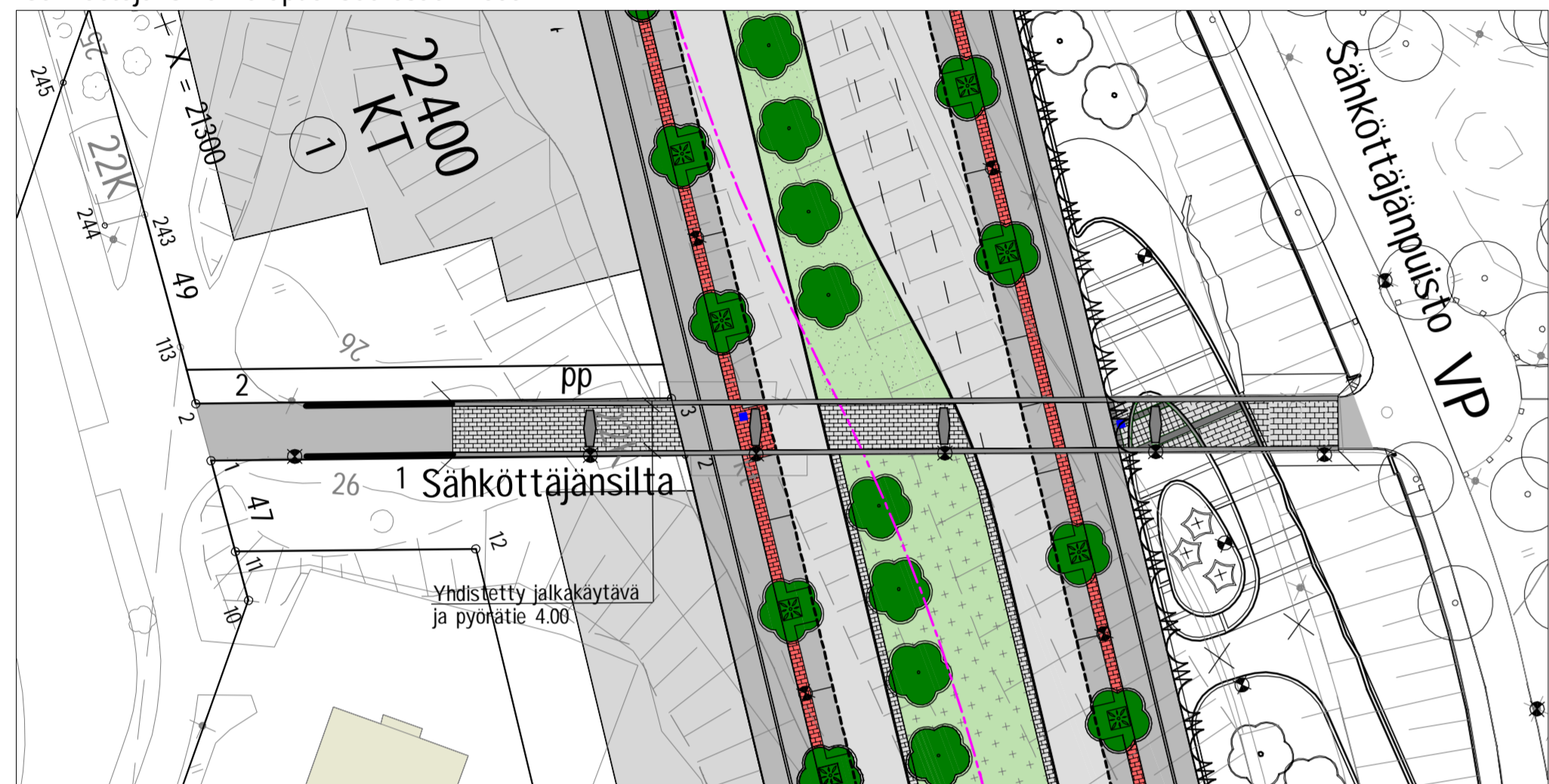
Sähkötäjänsillan alapuoliset osat 1:500
